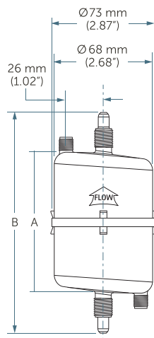
2.5" Disposable, Ø73 mm
