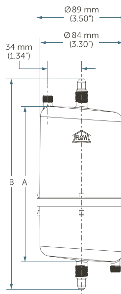
5" Disposable, Ø89 mm
