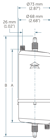
5" Disposable, Ø73 mm
