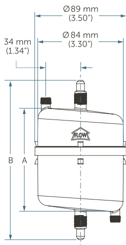
2.5" Disposable, Ø89 mm
